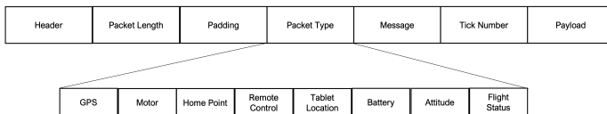
Fig. 2: Packet Structure of DJI DAT files
