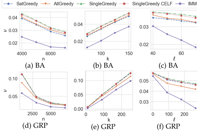
Fig. 2: RIM. BA ( n=5 \cdot 10^3 , \ell=50 , k=100 , \mu=2 ), GRP ( n=3 \cdot 10^3 , \ell=180 , k=90 ). W=0.1 , SatGreedy: \gamma=10^{-4} .
