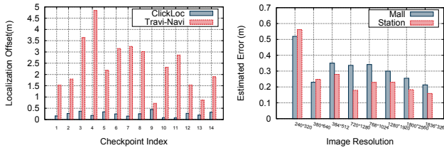
Figure 15. ClickLoc v.s. Travi-Navi
